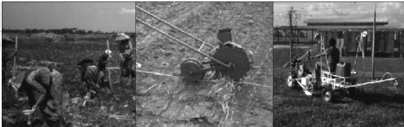
Figure 11 Trois exemples de méthodes de plantation sans préparation du sol: canne planteuse (photo de gauche), plantoir mécanique (photo du centre) et semoir automatique (photo de droite).
